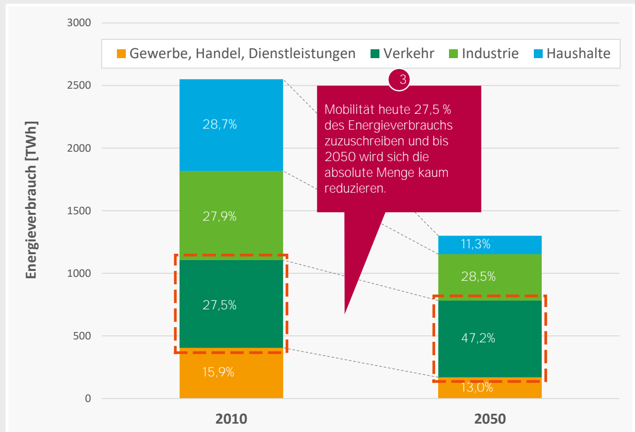
Vergleich des Energieverbrauchs in Deutschland von 2010 und 2050 je Sektor
